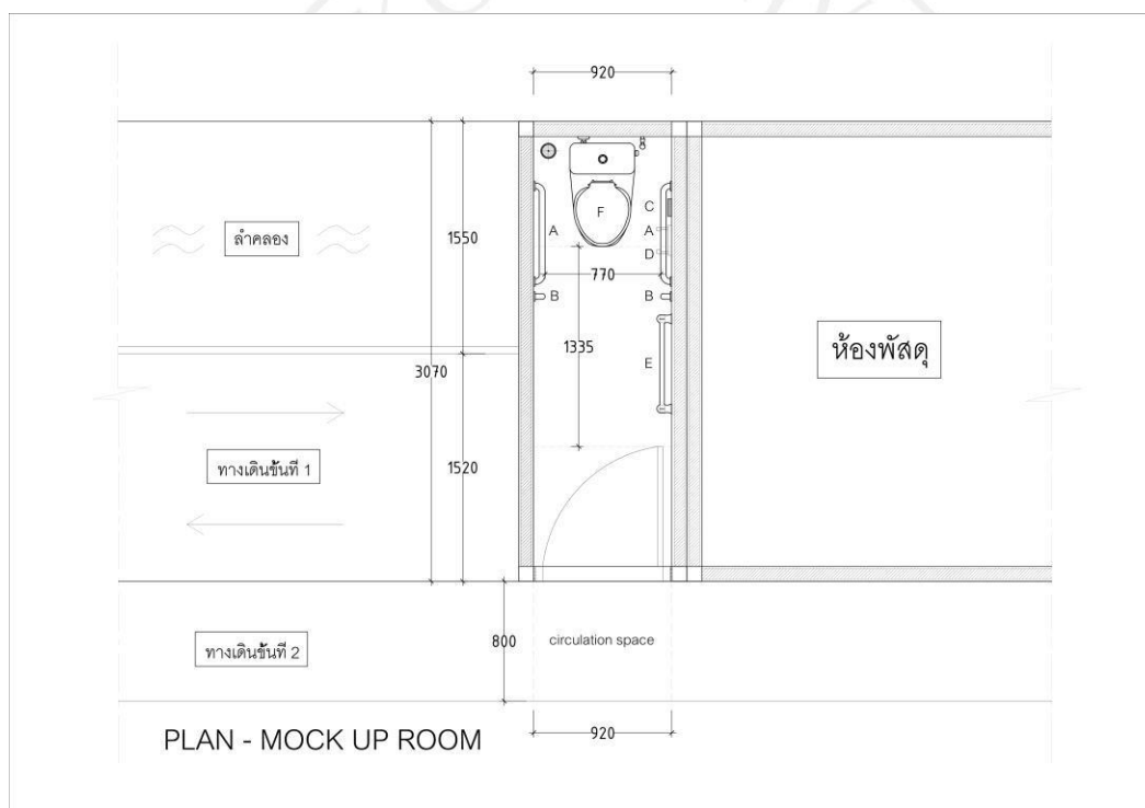
ภาพที่ 4.63: ตัวอย่างผังพื้นห้องนี้ ำ
