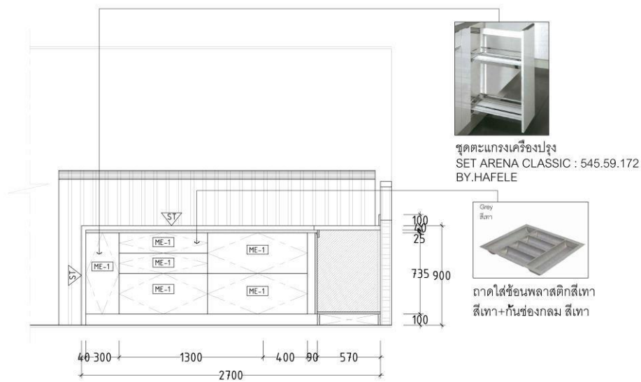
ELEVATION-A มัลติคัททำอิฐ
