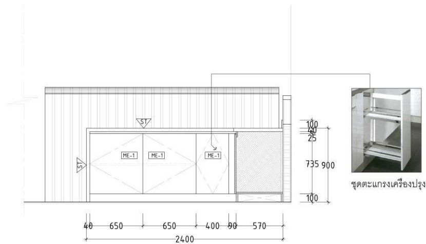
ELEVATION-A
