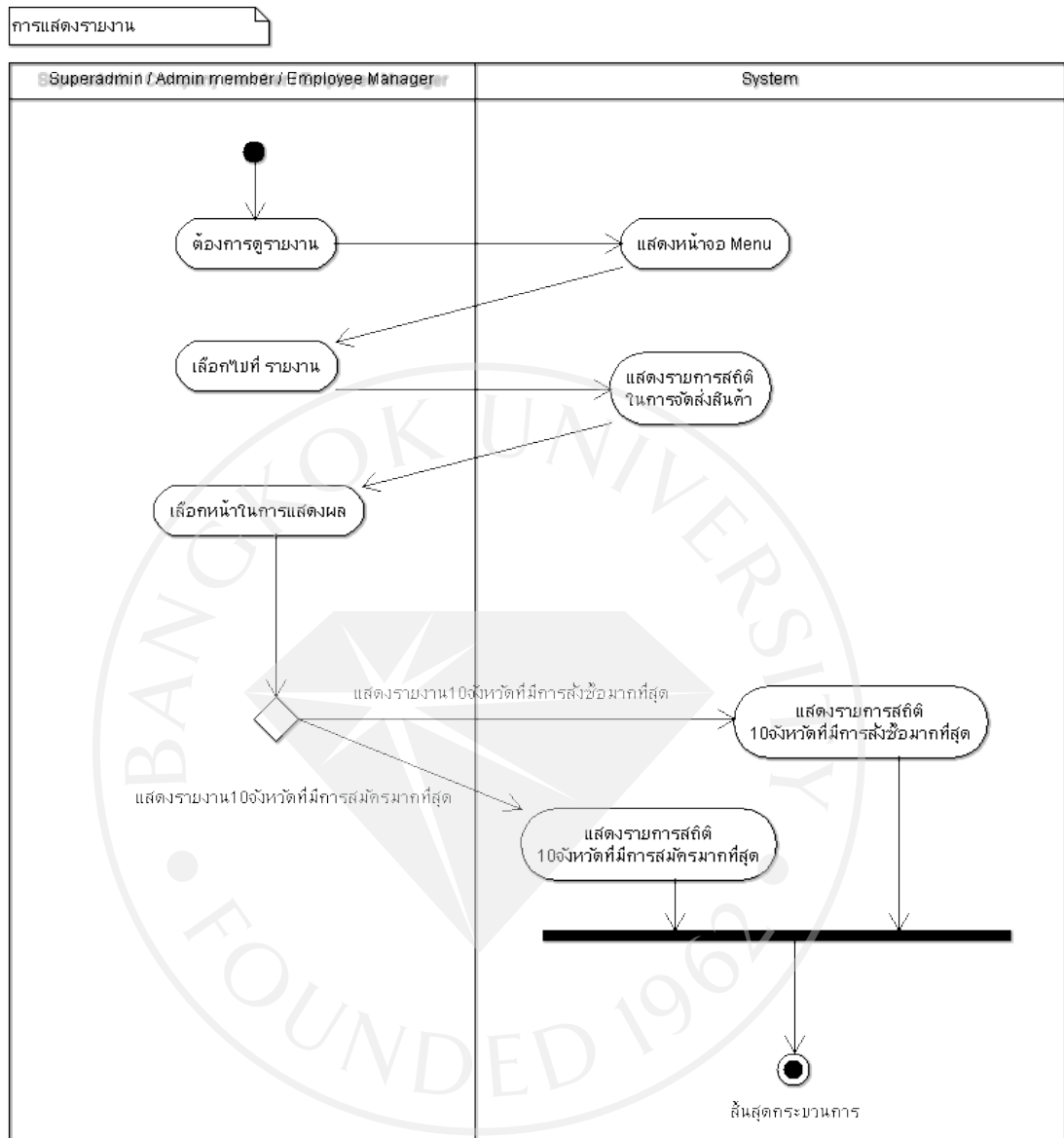
ภาพที่ 23: ขั้นตอนการแสดงผลรายงาน
