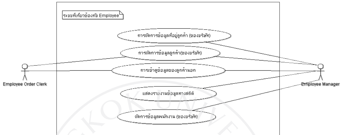
ภาพที่ 6: Use Case Diagram ฟังก์ชันที่เกี่ยวข้องกับพนักงาน
