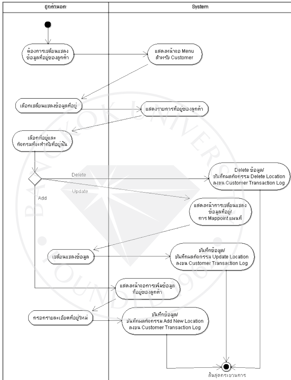
ภาพที่ 15: ขั้นตอนการเปลี่ยนแปลงข้อมูลที่อยู่ลูกค้าโดยลูกค้านอก
