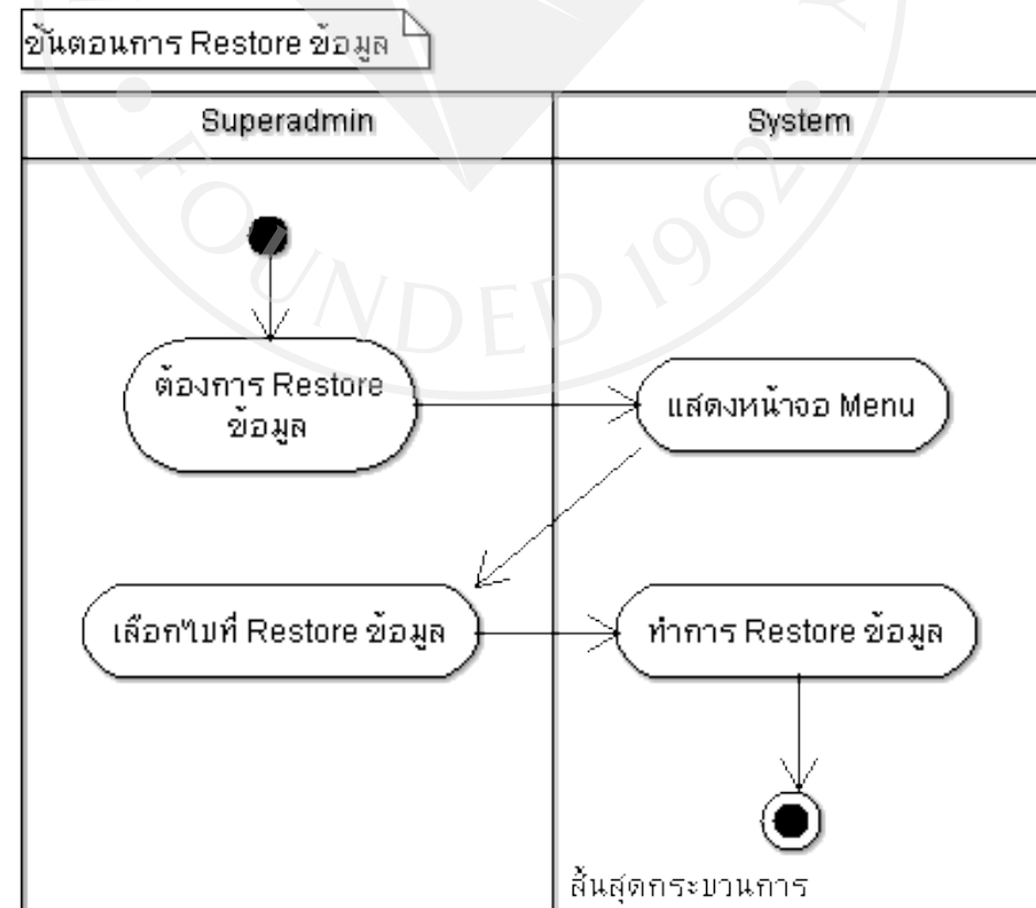
ภาพที่ 27 : ขั้นตอนการ Restore ข้อมูล
