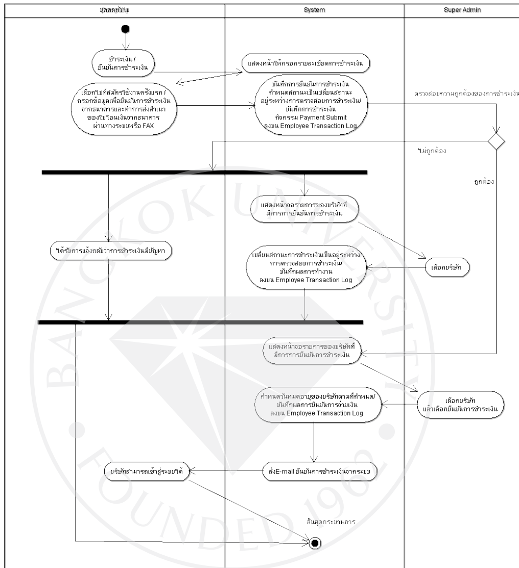
ภาพที่ 12: ขั้นตอนการยืนยันการชำระเงิน
