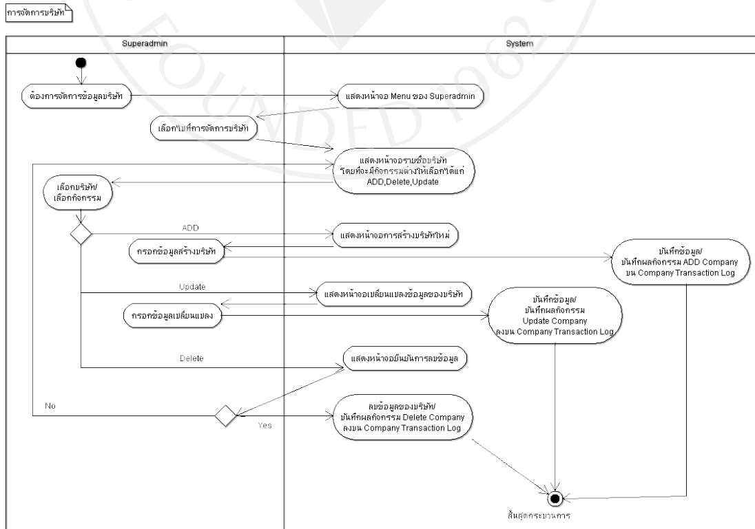
ภาพที่ 25: ขั้นตอนการจัดการกับบริษัท
