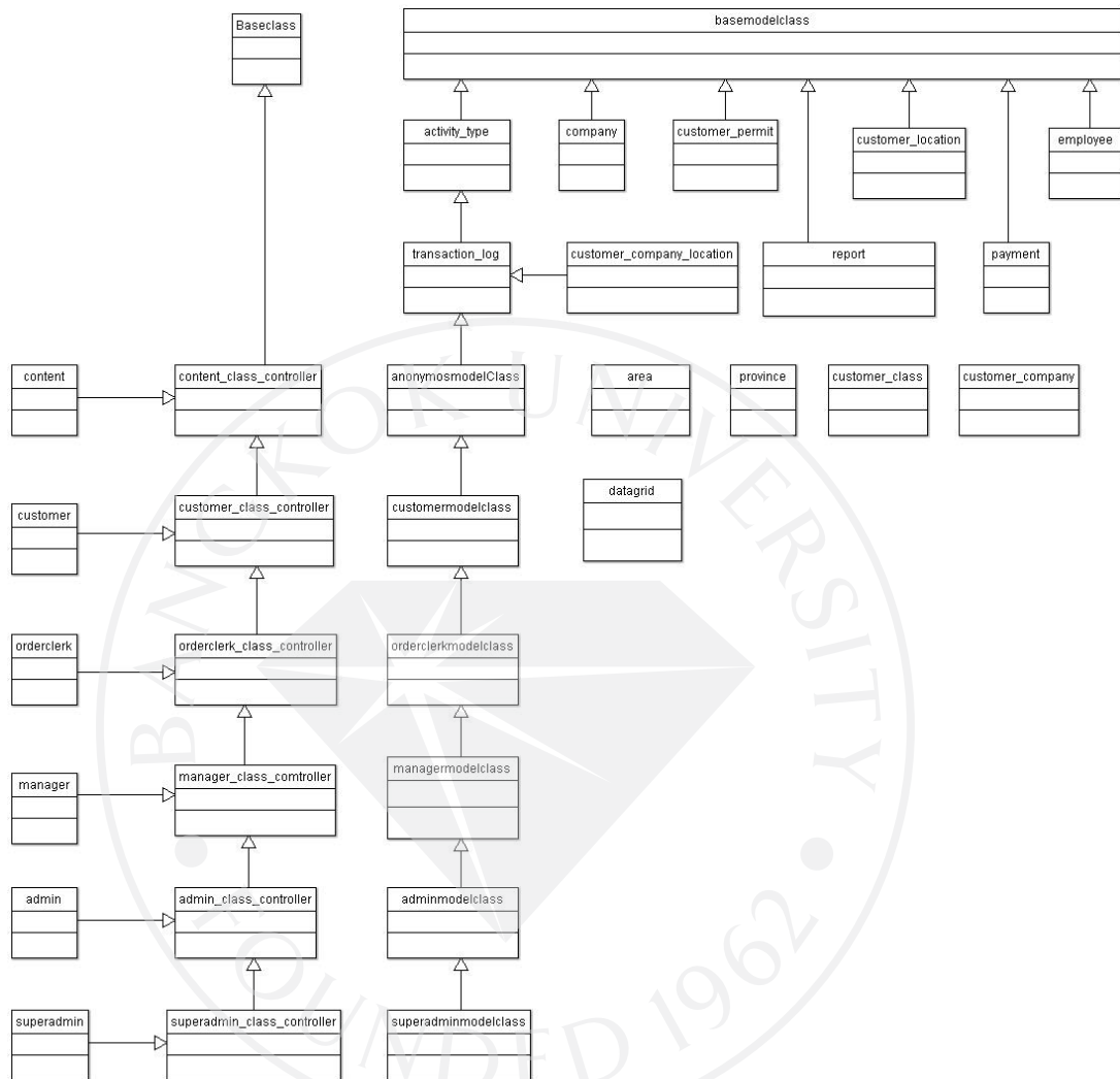
ภาพที่ 28: Class Diagram
