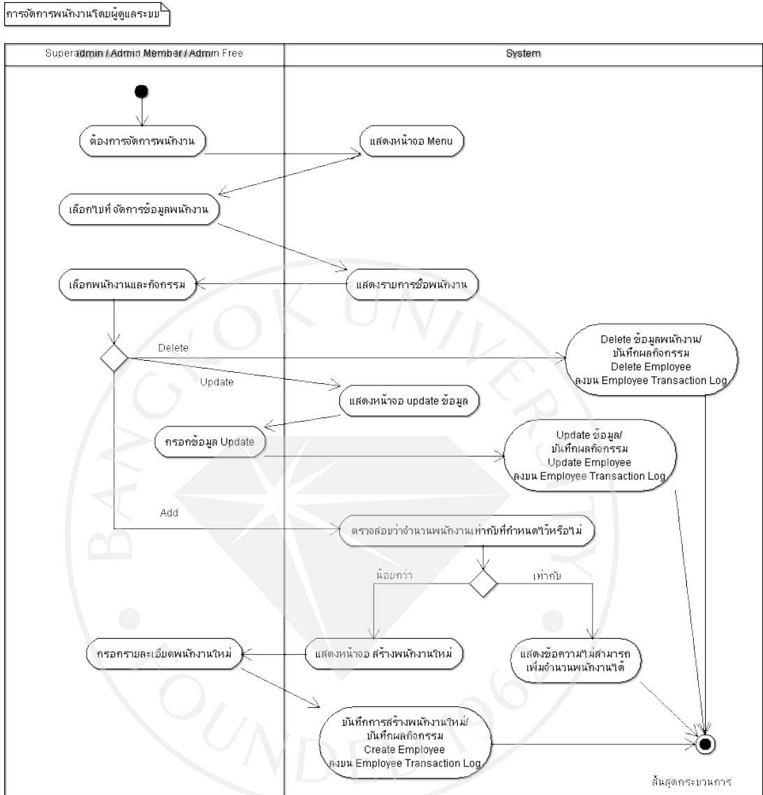
ภาพที่ 22: ขั้นตอนการจัดการพนักงานโดย Admin และ Super Admin
