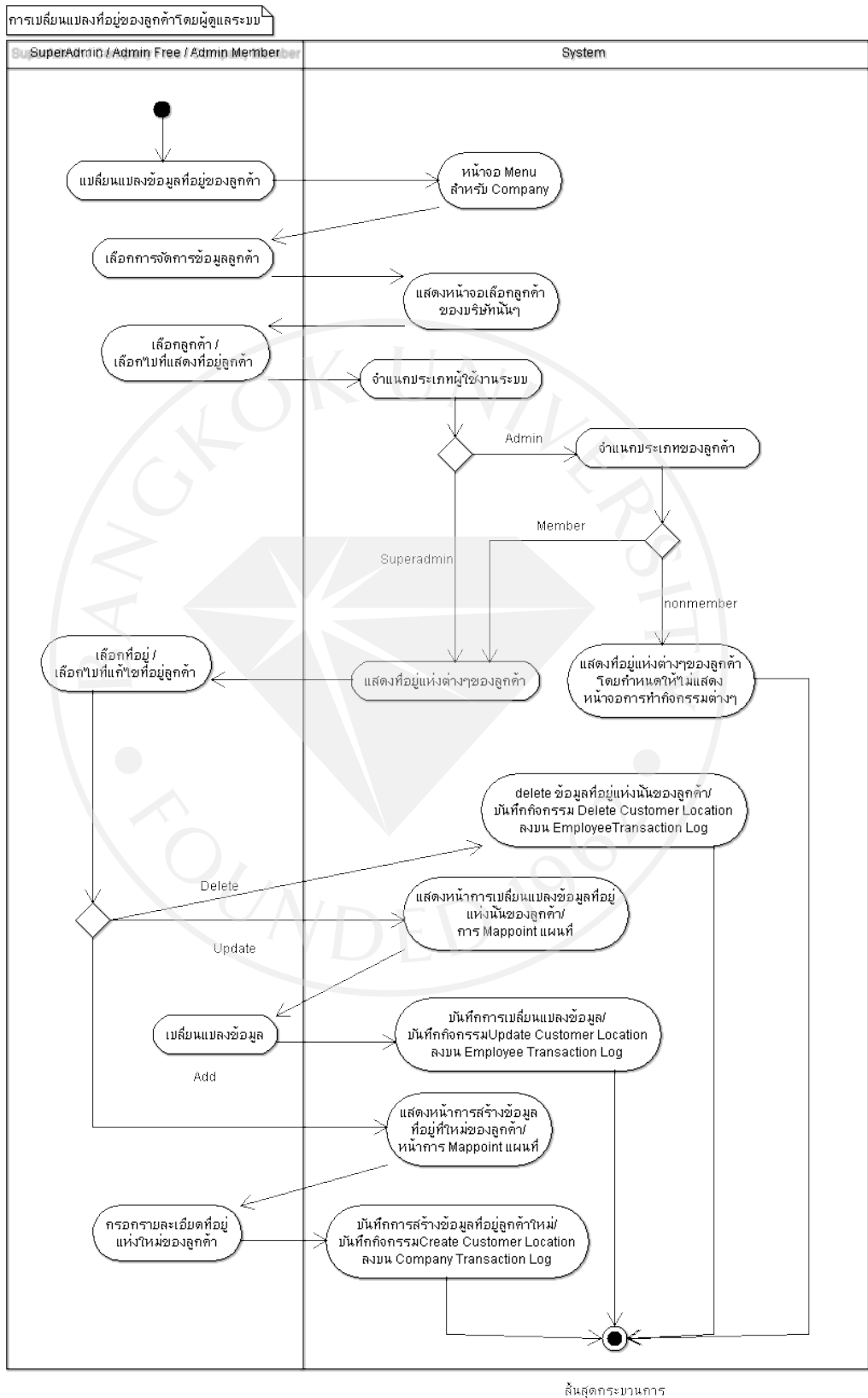
ภาพที่ 21: ขั้นตอนการจัดการข้อมูลที่อยู่ลูกค้าโดย Admin และ Super Admin
