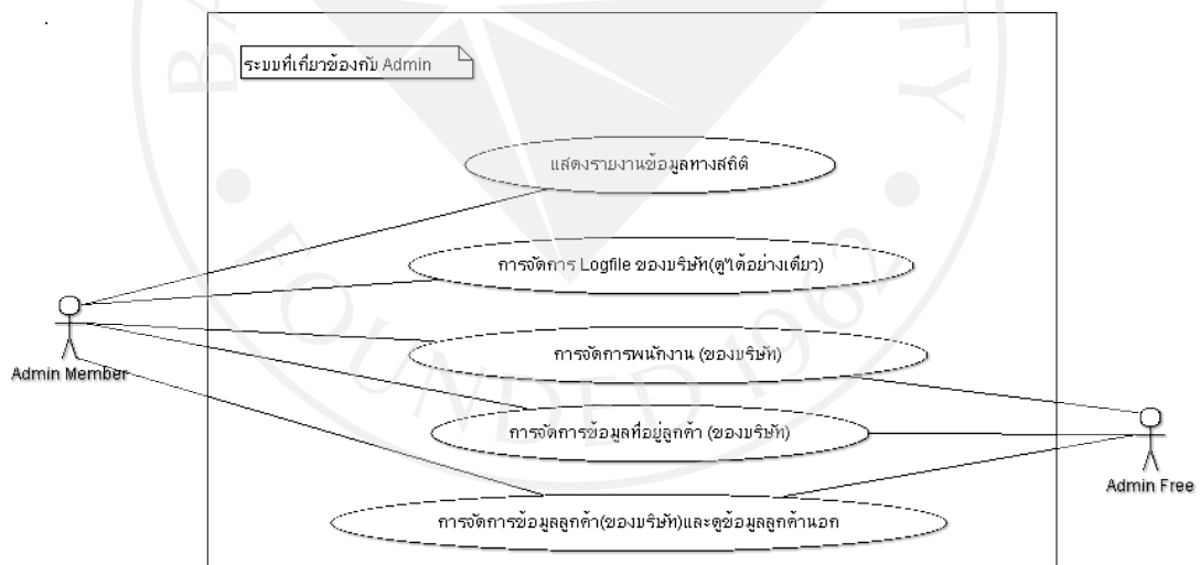
ภาพที่ 7: Use Case Diagram ฟังก์ชันที่เกี่ยวข้องกับ Admin
