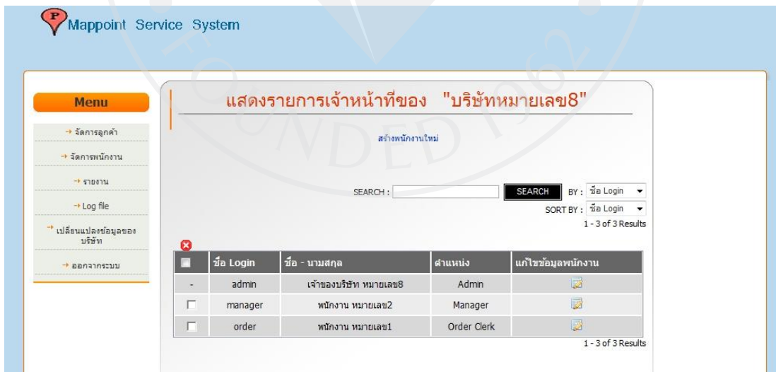
ภาพที่ 68: หน้าแสดงรายชื่อพนักงานในบริษัท สำหรับผู้ลงทะเบียนบริษัท
