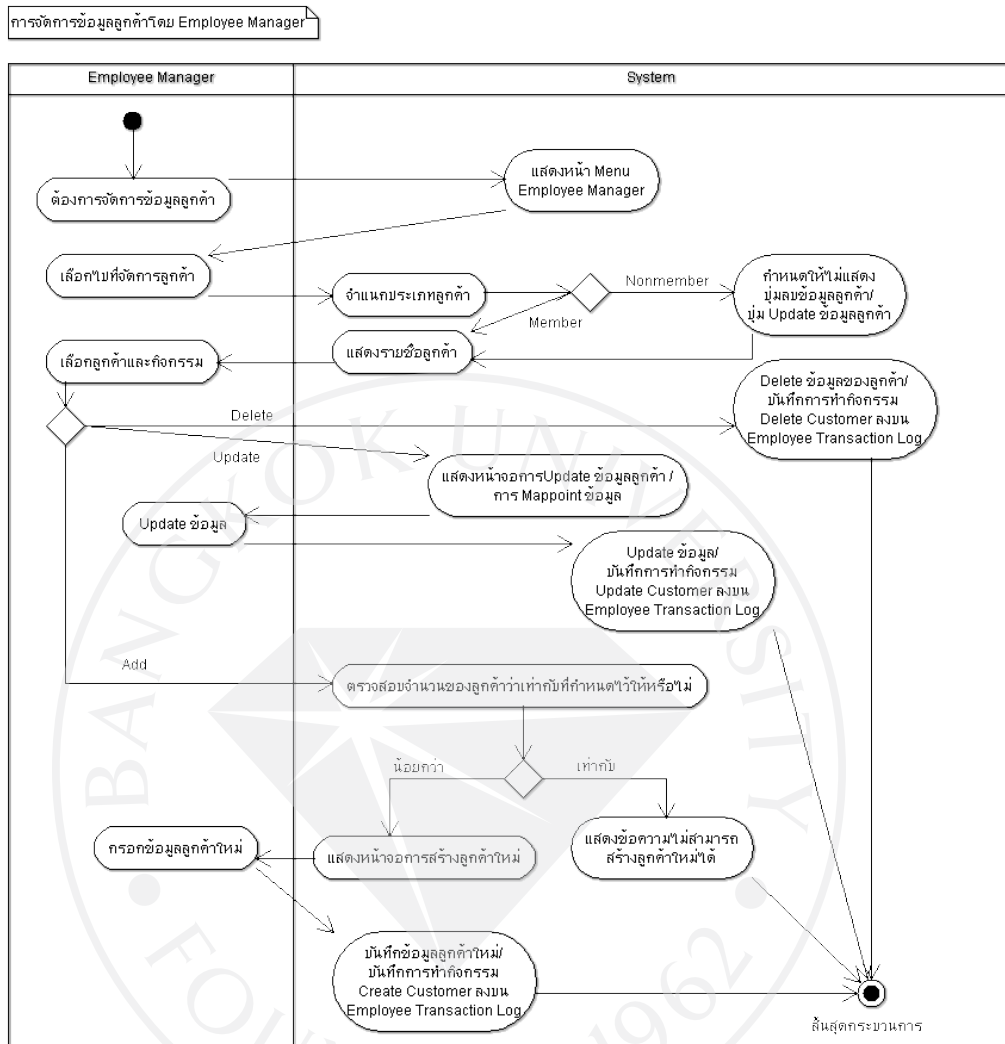
ภาพที่ 18: ขั้นตอนการจัดการข้อมูลลูกค้าโดย Manager
