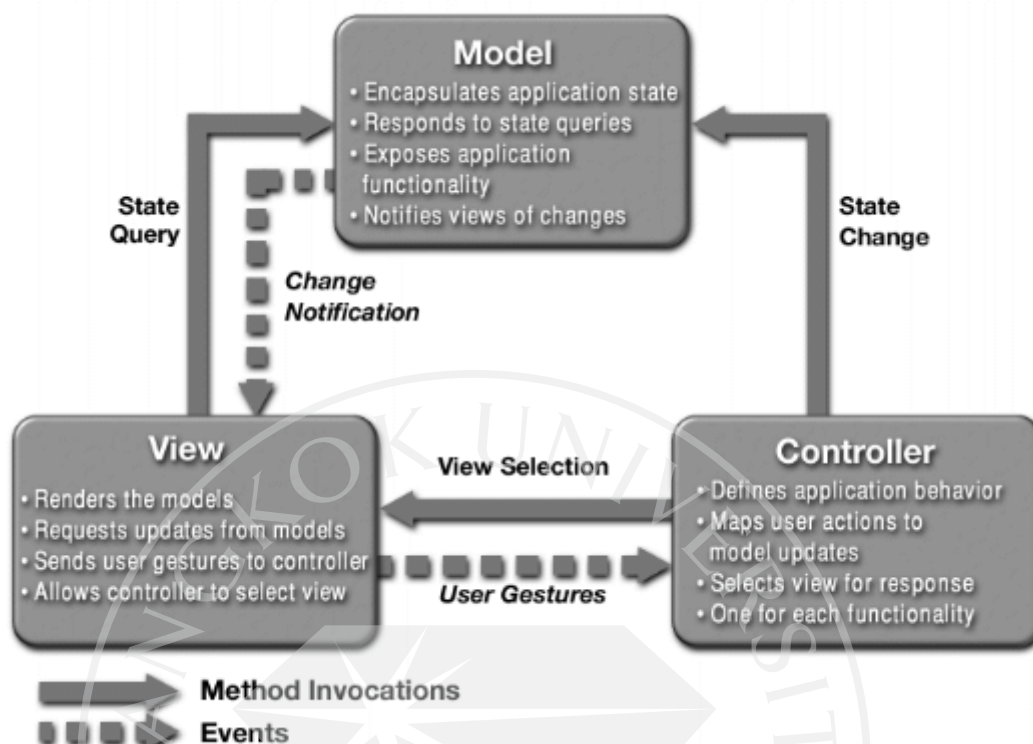
ภาพที่ 3: MVC Structure
