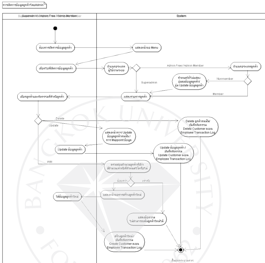
ภาพที่ 20: ขั้นตอนการจัดการข้อมูลลูกค้าโดย Admin และ Super Admin
